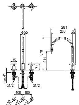
材質 真鍮 仕上 クロムメッキ (00)
