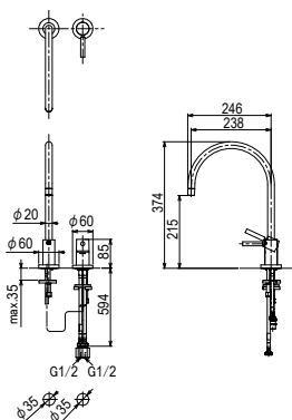
材質 真鍮 仕上 クロムメッキ (00)
