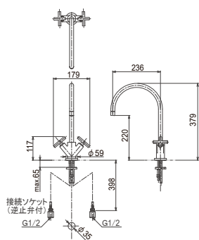
材質 真鍮 仕上 クロムメッキ (00)
