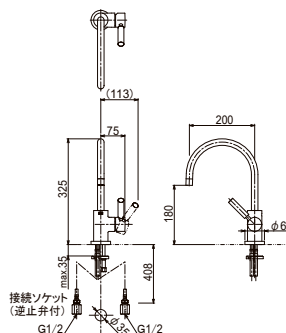
材質 真鍮 仕上 クロムメッキ (00)
