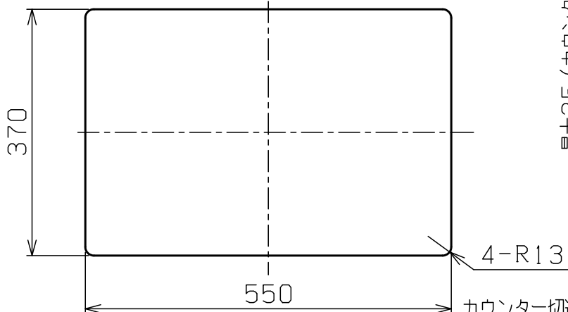
カウンター切込寸法図
