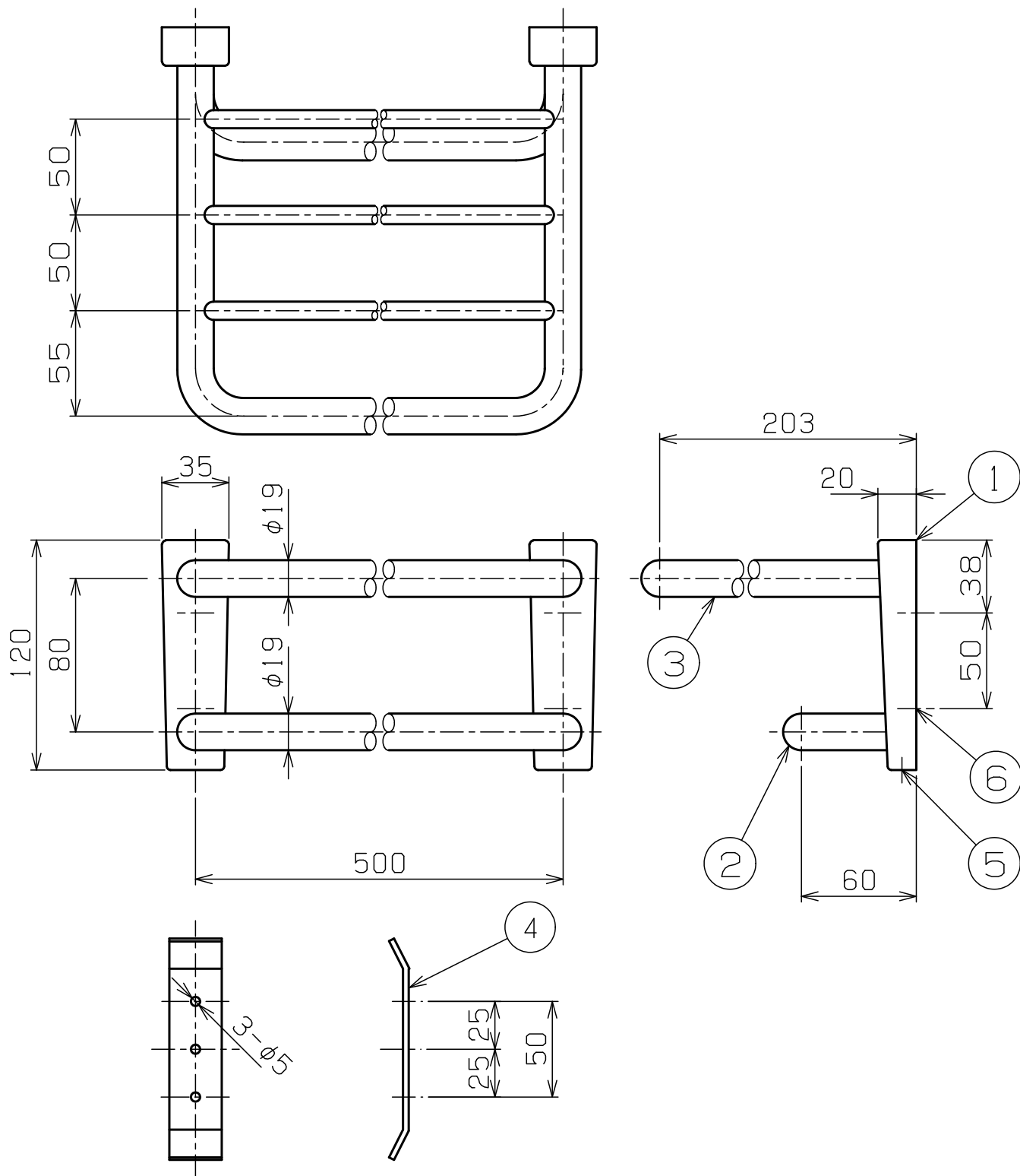
標準パイプ寸法 L-500m/m (特注サイズ250~500m/m以内受注生産可能)
